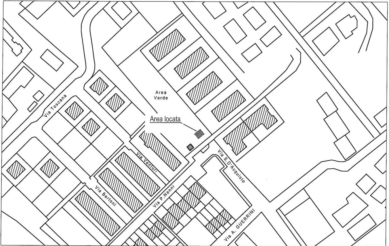
PARTICOLARE PLANIMETRIA - Scala 1:500
